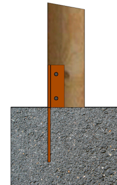
Pilar amb platina Pilar con pletina
